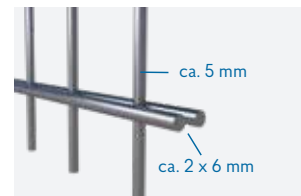
Typ „leicht“
